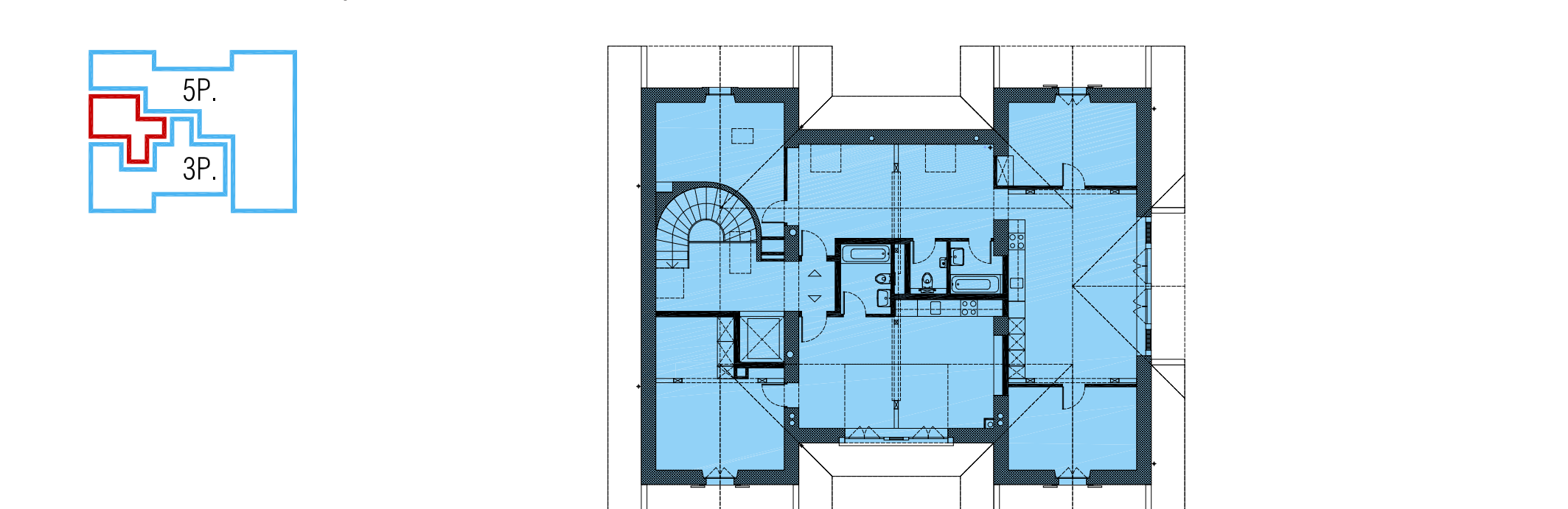
Plan des Combles / Mai
